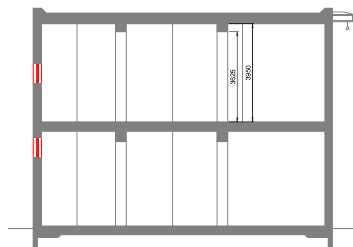
section D-D
